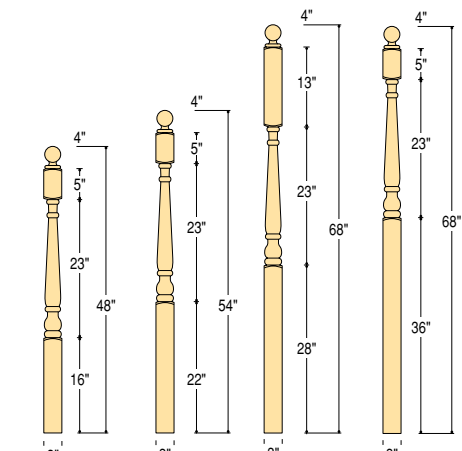
C-4540BT 3" Sq.
